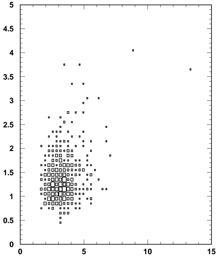
g218 (Gmax-Gmin)/Gmin.vs.RMS
