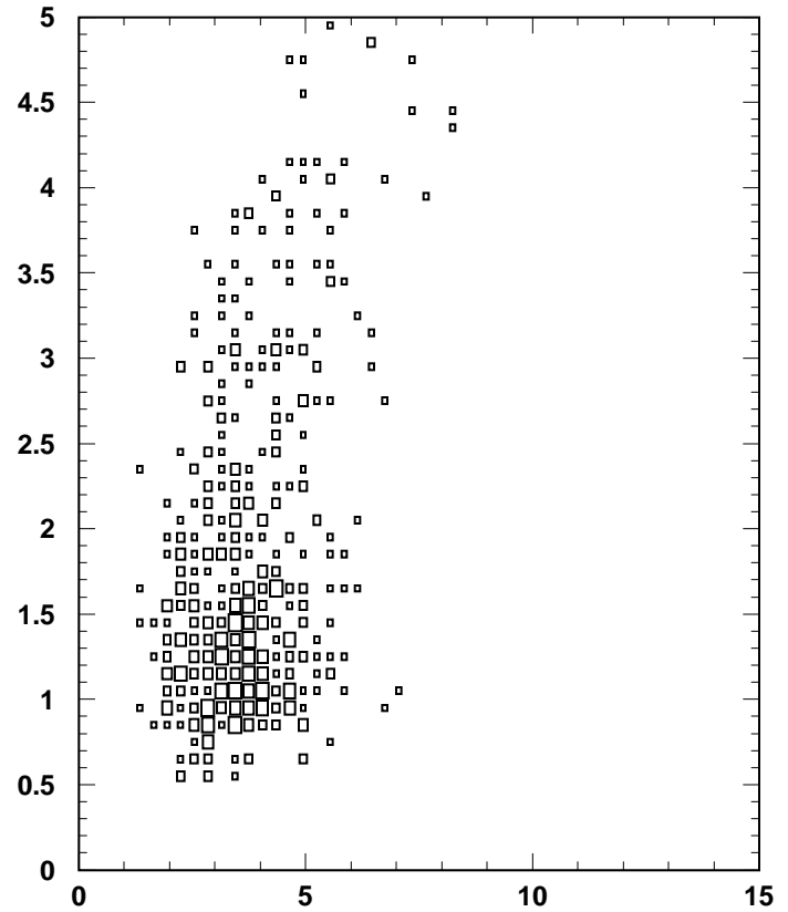
g225 (Gmax-Gmin)/Gmin.vs.RMS
